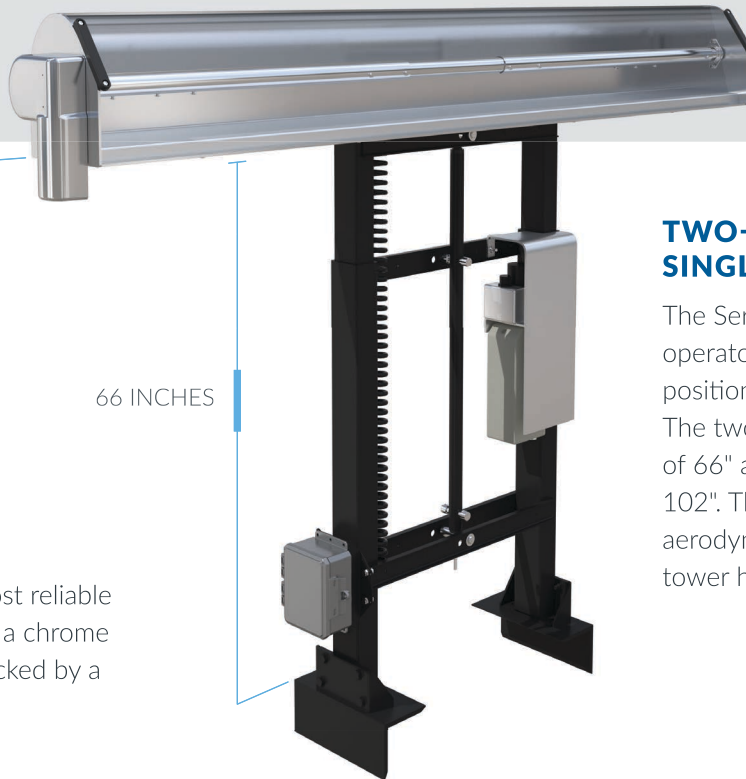
AeroForce 825 Fixed Pivot
